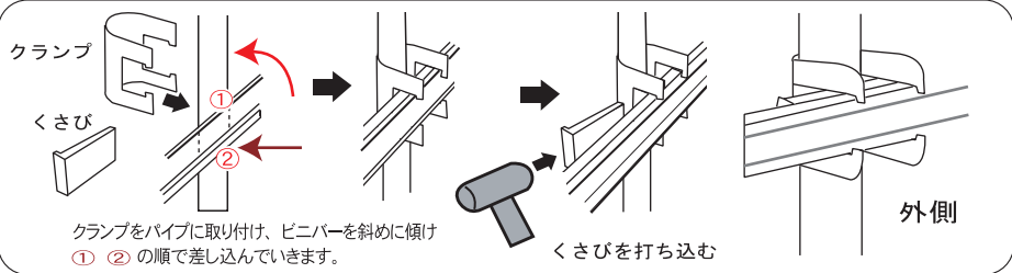
クランプと、ビニバーの取り付け方法
