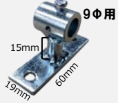
■ LB9 ブラケット 9φ用
