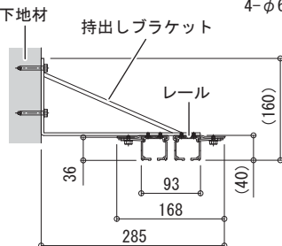
【B断面】
