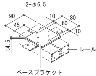
取り付け穴
