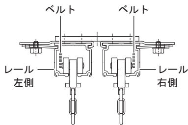
《レール側面図》 ※ベルト挿入側
