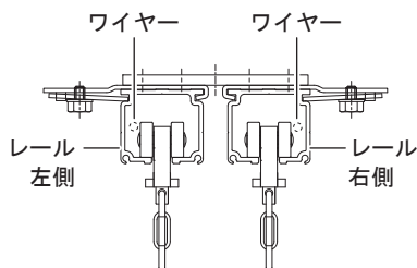
《レール側面図》 ※ワイヤー挿入側
