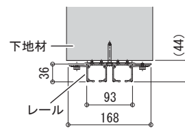
【A断面】
