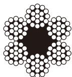
構成6×19 19本線6より中心繊維
