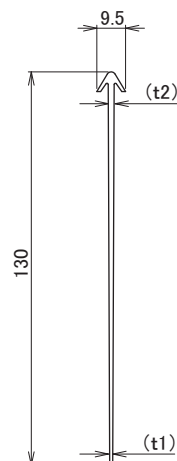
S-81 (レクト40/30 共通)
