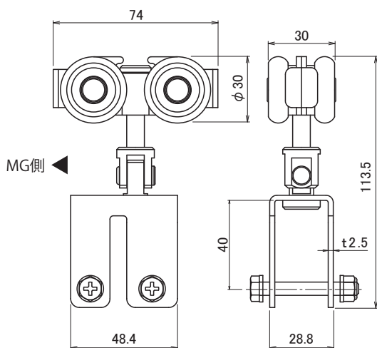
S-802D サイドポールストロング用 複車吊ランナー
