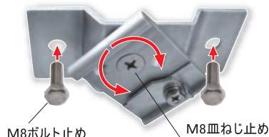
M8ボルト止め
