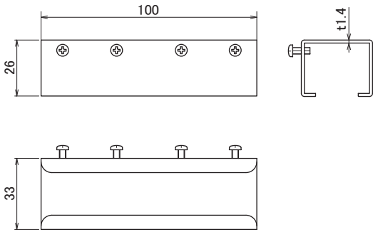
S-13 継力バー
