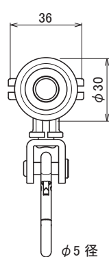
S-801C スナップランナー
