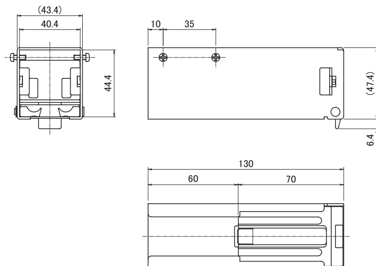
S-880 ラック入れエンドカバー
