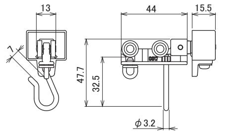
環下寸法 31mm
