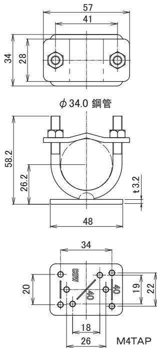
S-81 (レクト40/30 共通)
