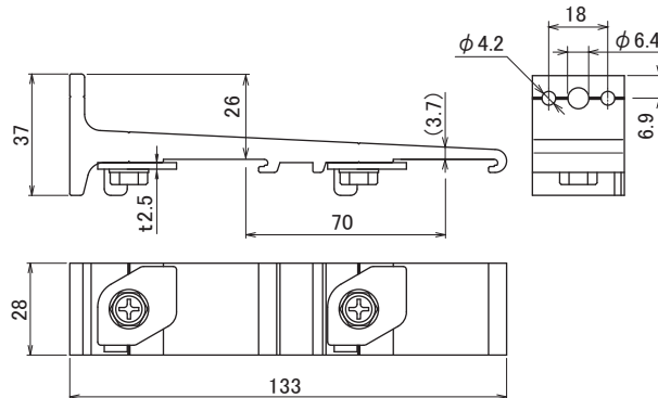
S-20WA アルミダブルブラケット
