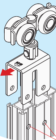
吊ランナー取付け方向図
