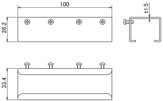
S-213 ステンレス継力バー
