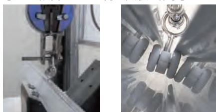
【レール傾斜 ランナー荷重試験の様子】
