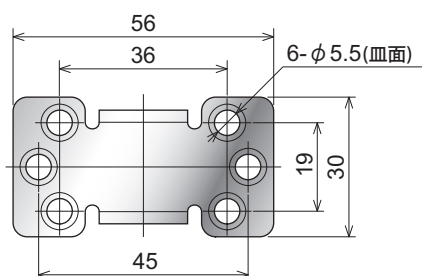
取付座寸法図
