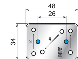
● 天井ブラケット取付位置
