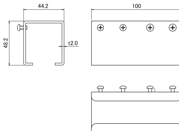
S-812 ステンレス継カバー
