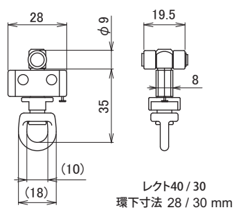
S-1PF (レクト40/30 共通)
