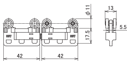
環下寸法 16mm
