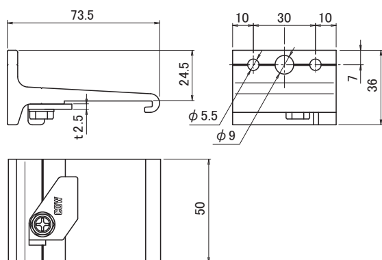
S-620A ブラケット
