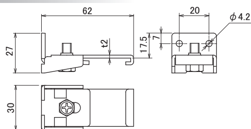
S-20 ブラケット
