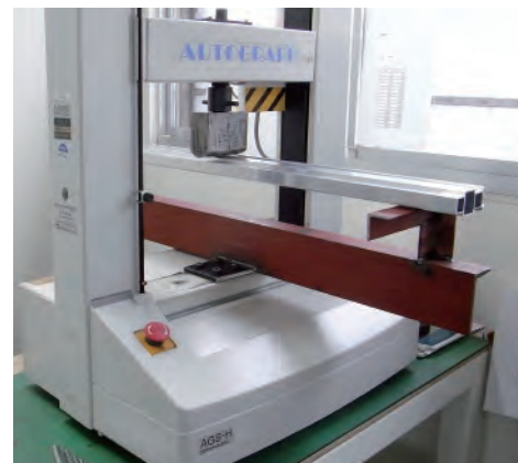
開閉ポールたわみ強度
