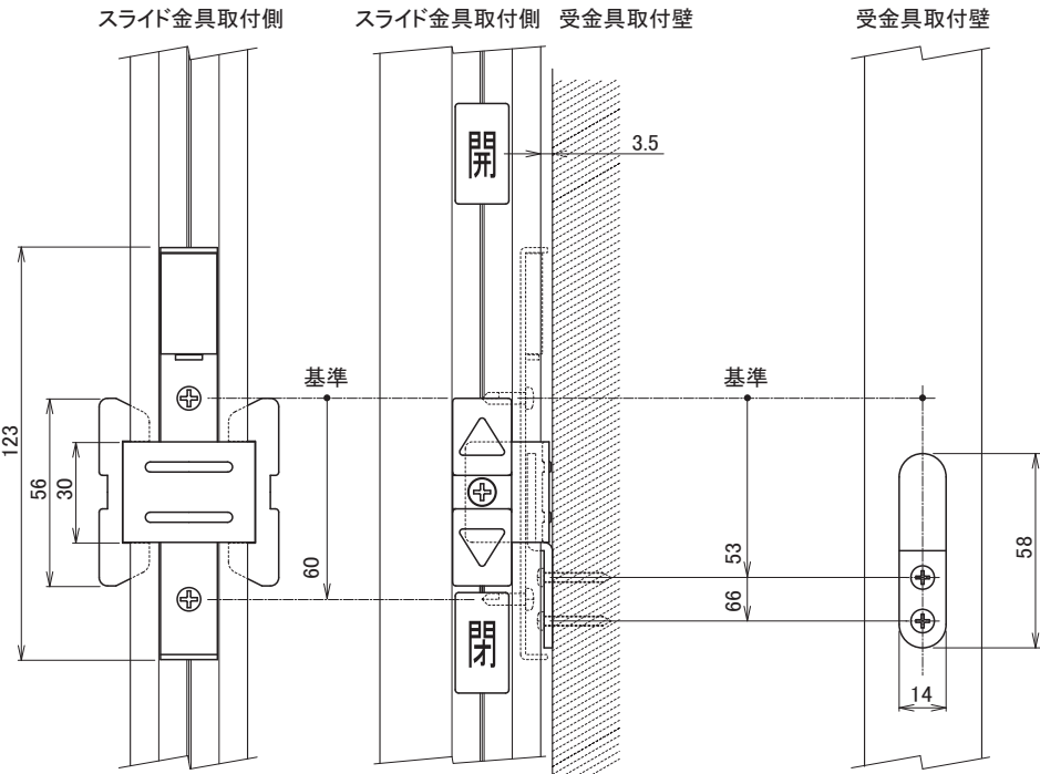
片開き時
