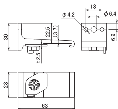
S-20A アルミブラケット
