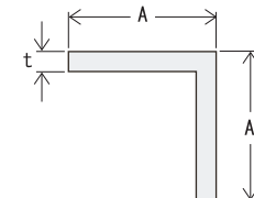
定尺:4000 mm 定尺販売品
