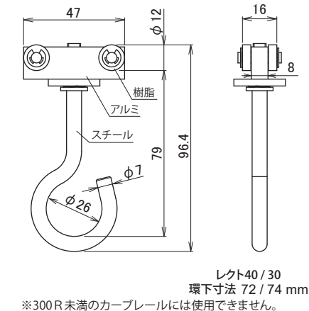
S-211 (アルトライン/レクト40/30 共通)
