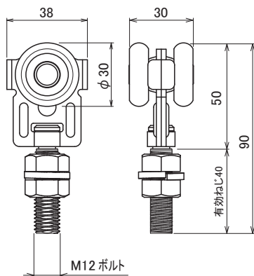
S-801B センターポールストロング用 ボルト式単車吊ランナー
