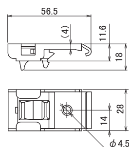
S-23T ワンタッチ天井ブラケット
