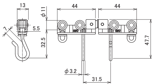
環下寸法 31mm
