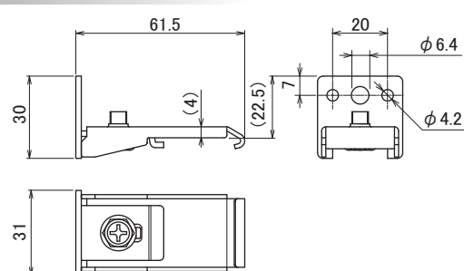
S-220 ステンレスブラケット
