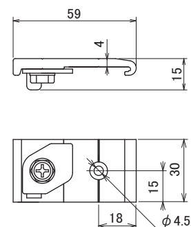
S-23A アルミ天井ブラケット
