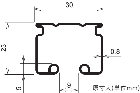
原寸大(単位mm)
