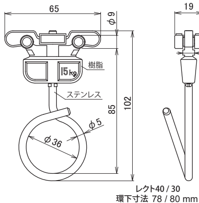
S-211 (アルトライン/レクト40/30 共通)
