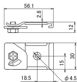
S-23 天井ブラケット
