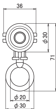
S-801A リングランナー
