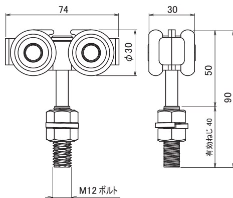
S-802B サイドポールストロング用 ボルト式複車吊ランナー
