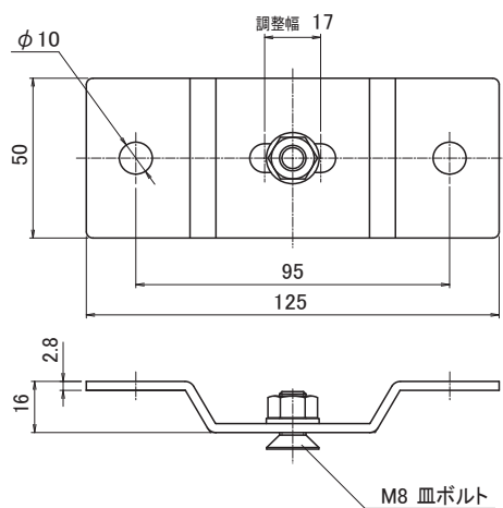
S-624 天井ブラケットアダプター
