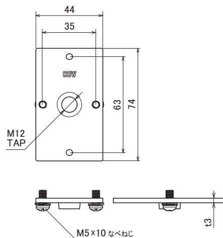
S-605 のれんシート用アタッチメント
