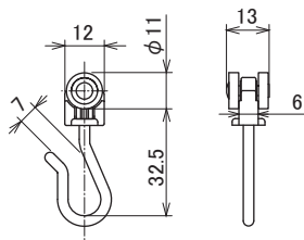
環下寸法 31mm
