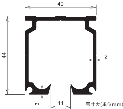
取付寸法図 (単位mm)
