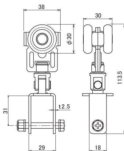
S-801D センターポールストロング用 単車吊ランナー
