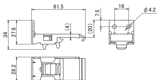
S-20T ワンタッチブラケット
