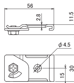
S-223 ステンレス天井ブラケット
