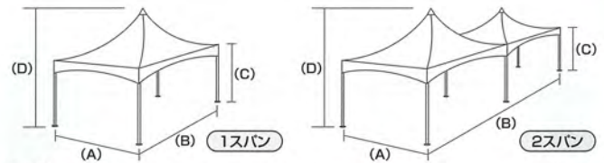
〔外寸法図〕
