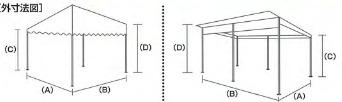
〔外寸法図〕
