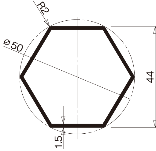
アルミ合金番号 : 6061T-6 サイズ : アルミ六角パイプ 44mm×1.5mm 厚
