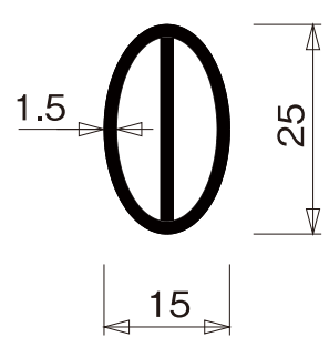
アルミ合金番号 : 6061T-6 サイズ : アルミ精円パイプ 15mm×25mm×1.5mm 厚
