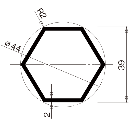
アルミ合金番号 : 6061T-6 サイズ : アルミ六角パイプ 39mm×2.0mm 厚
