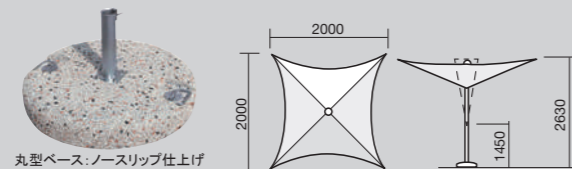
丸型ベース：ノースリップ仕上げ
