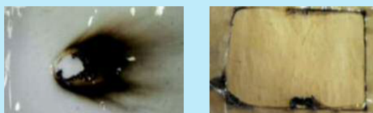
2分燃焼試験後の防災フィルム(左)と一般フィルム(右)
