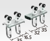
D30マグネットランナー(両開) ワンタッチランナータイプ
