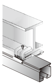
Bタイプ(鋼材の下)
