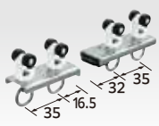
D30マグネットランナー(両開) 通常ランナータイプ
