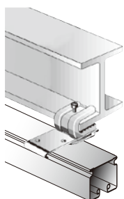
Aタイプ(鋼材から持出し)
