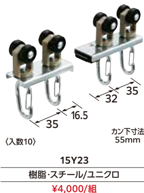
D40マグネットランナー(両開) ワンタッチランナーAタイプ
