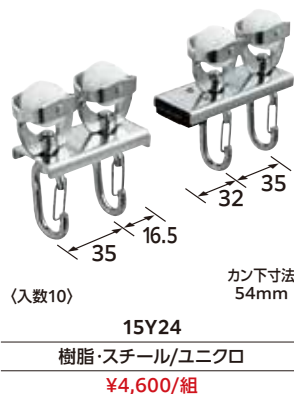
D40マグネットランナー(両開) ワンタッチランナーSタイプ
