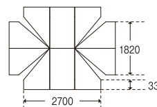
天幕(平面図)
