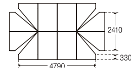
天幕(平面図)
