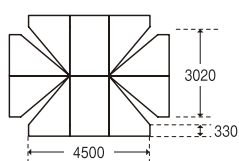
天幕(平面図)
