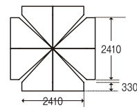
天幕(平面図)
