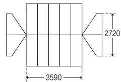
天幕(平面図)
