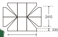
天幕(平面図)
