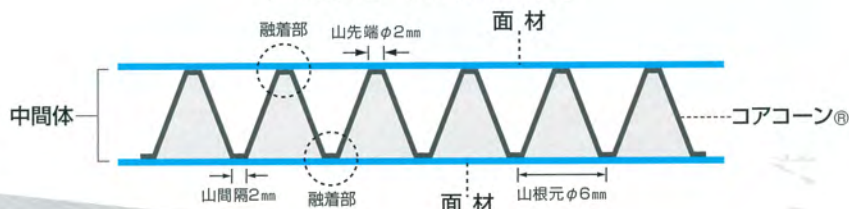
【シングルコーン®の基本構成】
