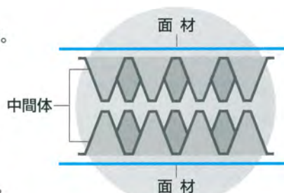
溶着前の4層構造
