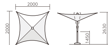
丸型ベース:ノースリップ仕上げ
