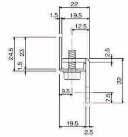
● カーブレール
