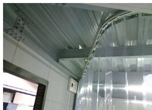
●シート：オーロラ帯電防止透明 100w カーブレール
