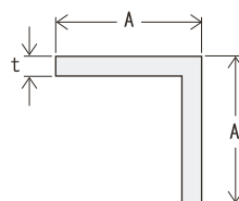
定尺:4000 mm 定尺販売品
