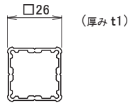
MRCA センターポール アルファ
