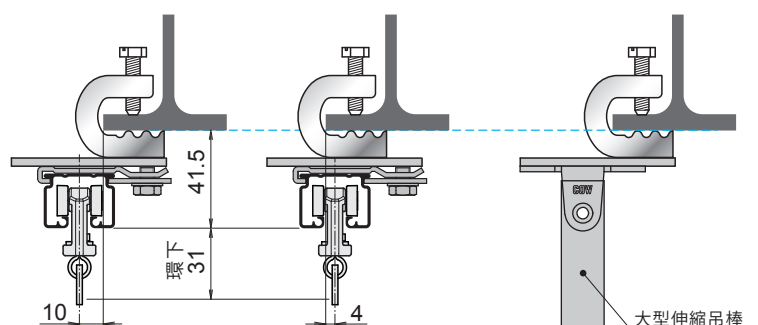
大型伸縮吊棒
