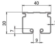
KH スチールレール
