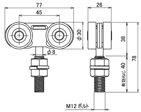
S-602B 複車ボルトランナー
