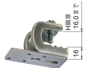
クランプ付 ブラケットベースM
