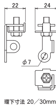
S-204 ステンレスフリーストップ
