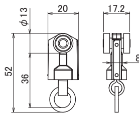
S-5A 重量級オールステンレスランナー (ベアリング)
