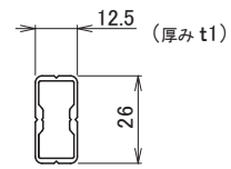
MRE センターポール スリム
