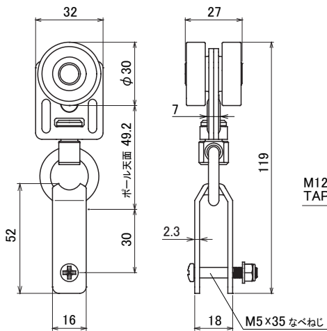
S-601AD ポール吊金具付きランナー
