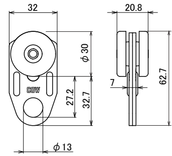
S-6T トロリーランナー
