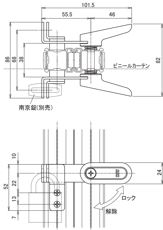
MR-27 サイドポール ライト用 両開きロック金具
