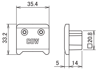
MR-33 サイドポール アルファ用 エンドキャップ
