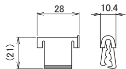
S-83 (レクト40/30共通)
