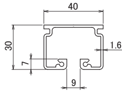
KT アルミレール
