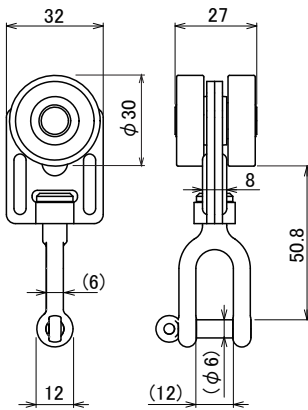
S-601C シャックルランナー
