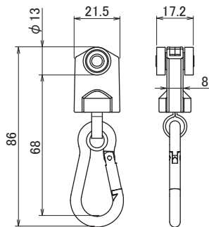
S-2C 重量級スナップランナー (ベアリング)
