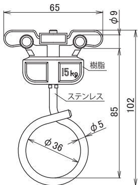
S-42 (レクト40/30 共通)
