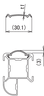
MR-2 サイドクッション
