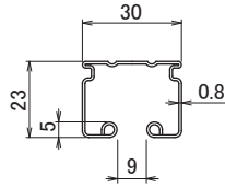
S-3A/S-7A ランナー
