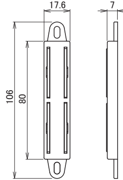
MR-3 マグネット
