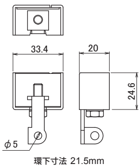
S-22A/S-222 吊ブラケット/ステンレス吊ブラケット
