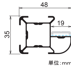
MRSA アルミ押出材 A6063S-T5 アルマイト+クリア塗装仕上げ
