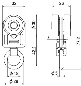
S-601A ランナー
