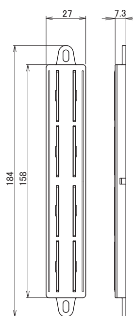
MR-3L ロングマグネット
