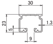
KS アルミレール
