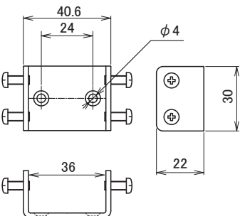
MR-10 ポール固定金具
