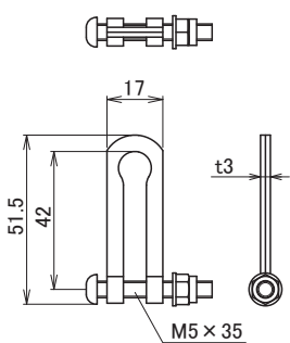
MR-10 ポール固定金具
