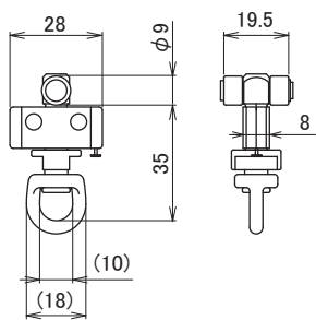
S-1PF (レクト40/30 共通)
