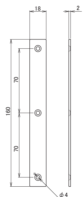
MR-4L ロングマグネット受座
