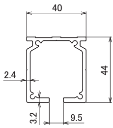
KV アルトラックレール
