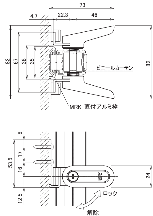
MR-28 サイドポール ライト用 片開きロック金具
