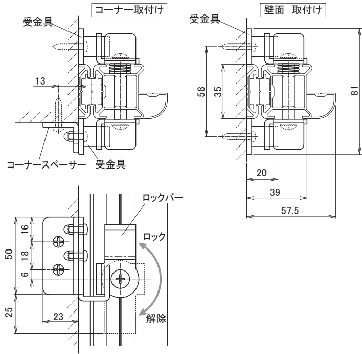
MR-9K サイドポール アルファ用 片開きロック金具 (MBタイプ)
