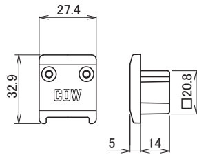
MR-34 サイドポール ライト用 エンドキャップ
