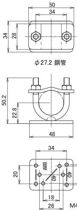
S-81 (レクト40/30共通)
