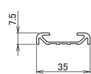
MRK 直付アルミ枠
