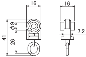
S-1 ランナー
