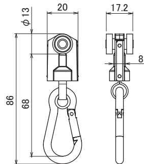
S-5C 重量級オールステンレススナップランナー (ベアリング)
