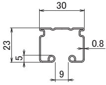
S-1 ランナー
