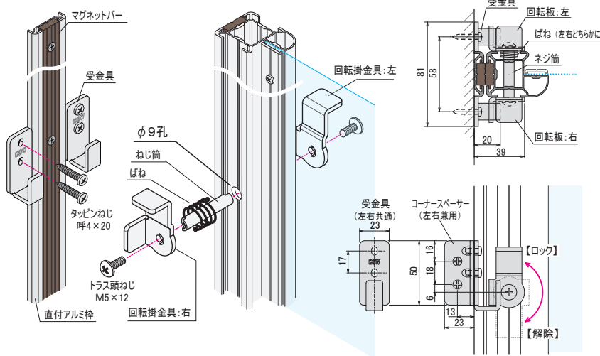
マグネットバー + サイドポール アルファ
