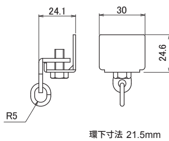
S-39 エンドストップ
