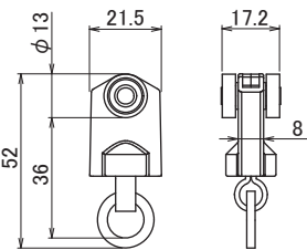
S-2A 重量級ランナー (ベアリング)
