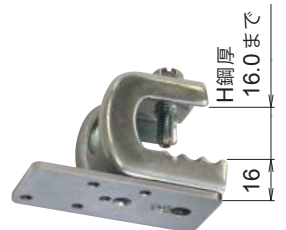
クランプ付 ブラケットベースM
