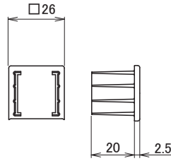
MR-5CP センターポール アルファ用 エンドキャップ
