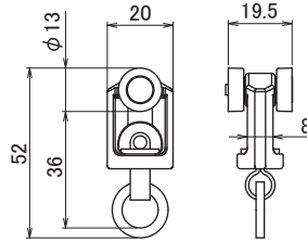
S-3A/S-7A ランナー
