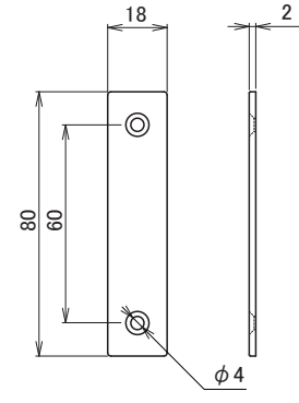
MR-4 マグネット受座
