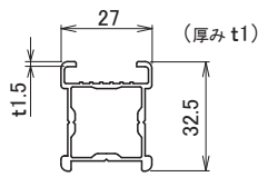
MRSL サイドポール ライト
