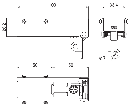
S-80 ラック入れエンドカバー
