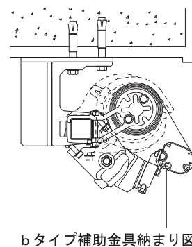
b タイプ補助金具納まり図
