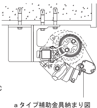
a タイプ補助金具納まり図
