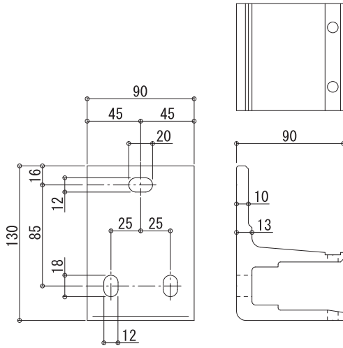
[1] 壁付用取付ブラケット
