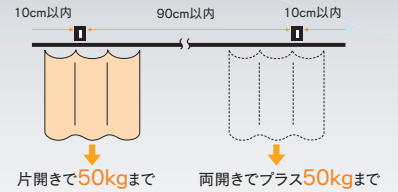
D40ブラケット取付間隔とカーテン適正重量表
