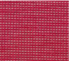
CK25 red レッド 透光率 24% Mansel value(マンセル値) 紫外線カット率 78% (H)0.89R(V)4.67(C)7.87
