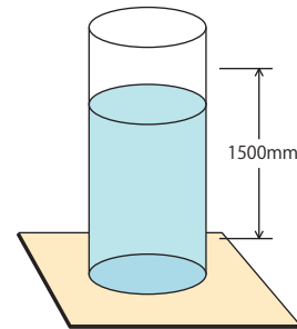
（図8）耐水試験の原理 上記試験で水準装置が1500mm高の時の水圧は、生地の上に円筒を固定して水を注いでいき、水位が1500mmになった時に生地にかかる水位とひとしい。
