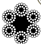
構成6×24 24本線6より中心および 各ストランド中心繊維
